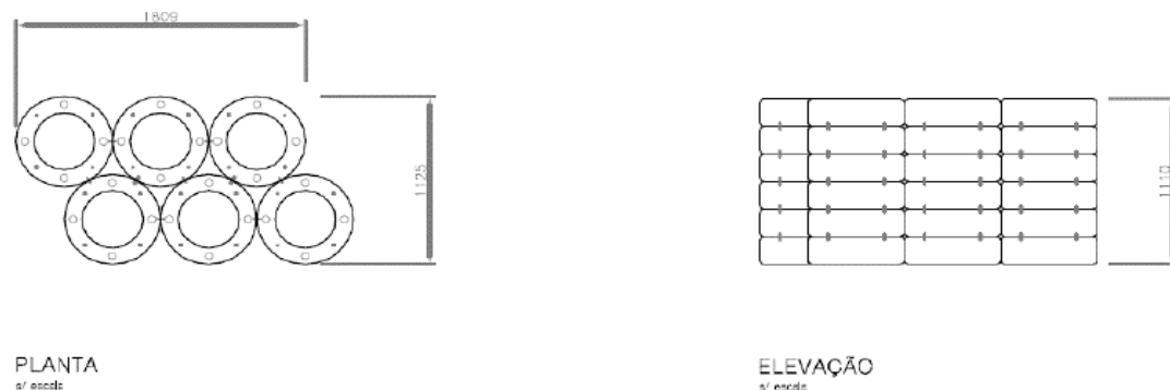
Figura 7 - Detalhamento do Módulo de Barreira de Pneus
