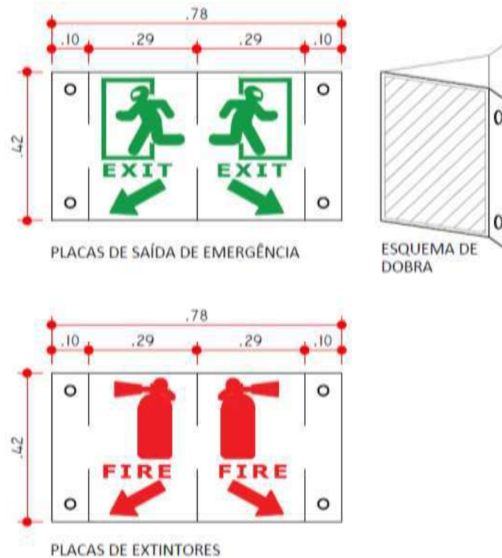
Figura 4 – Placas de Sinalização de Saída de Emergência e Extintores com indicativo de esquema de dobra
