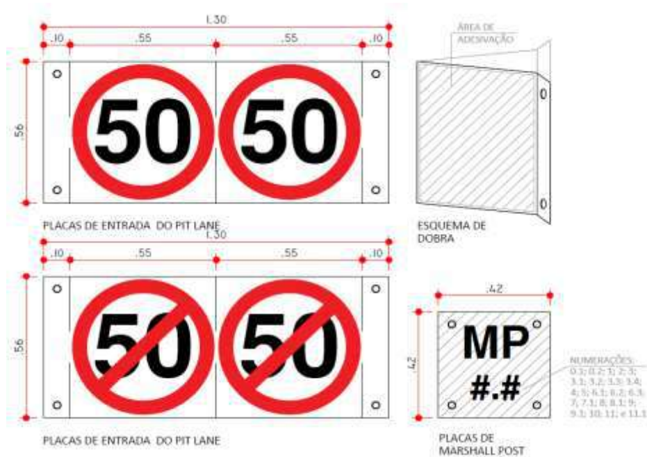
Figura 5 – Placas de Entrada do Pit Lan com indicativo de esquema de dobra e Placa de Postos Marshall.
