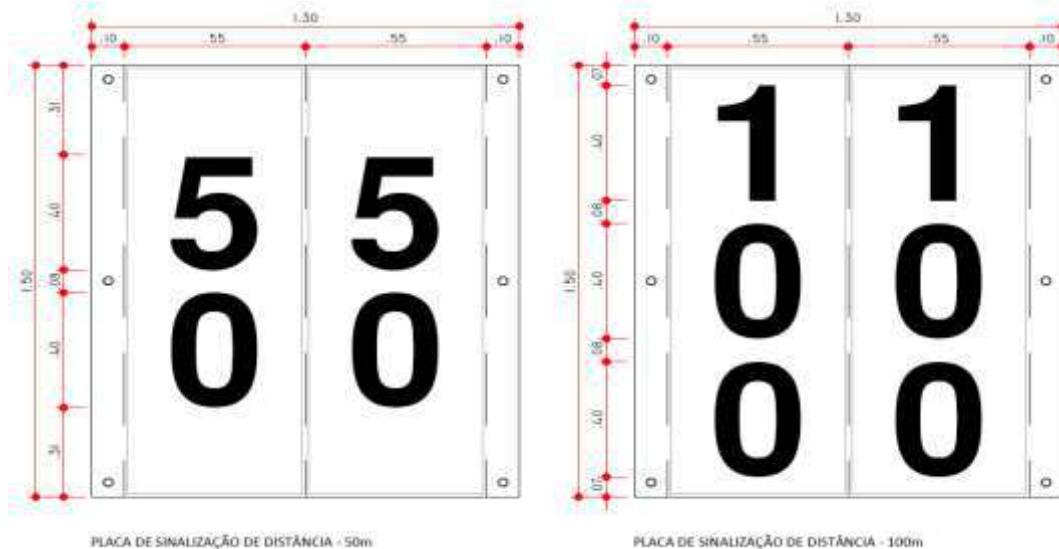
Figura 6 – Placas de Sinalização de distância
