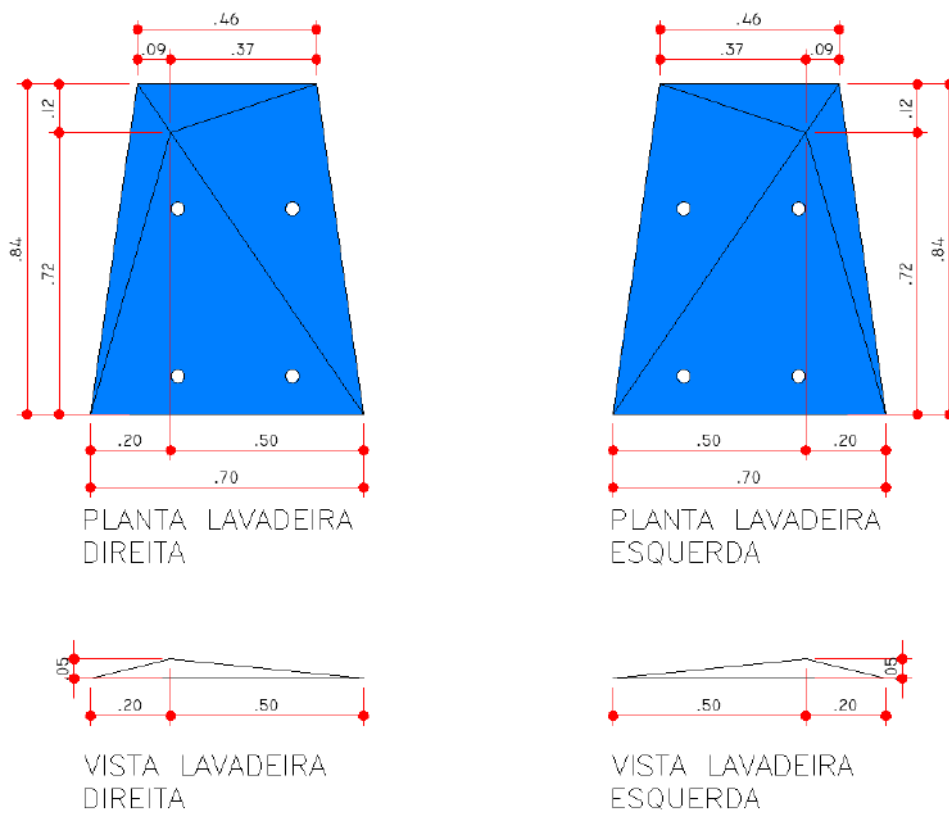
Figura 6 - Lavadeira metálica
