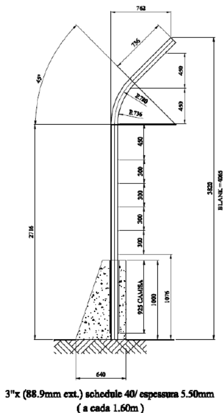
Figura 2 - Detalhamento das estruturas verticais para o gradil de proteção alto.
