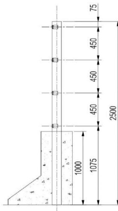
Figura 1 - Detalhamento das estruturas verticais para o gradil de proteção baixa.
